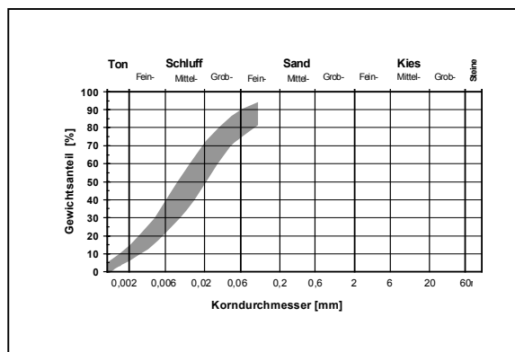
Abb. 10 : Baggerabschnitt 4, Körnungsband Klei (3 Proben)
