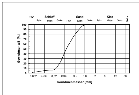
Abb. 20 : Baggerabschnitt 9, Körnungslinie Klei
