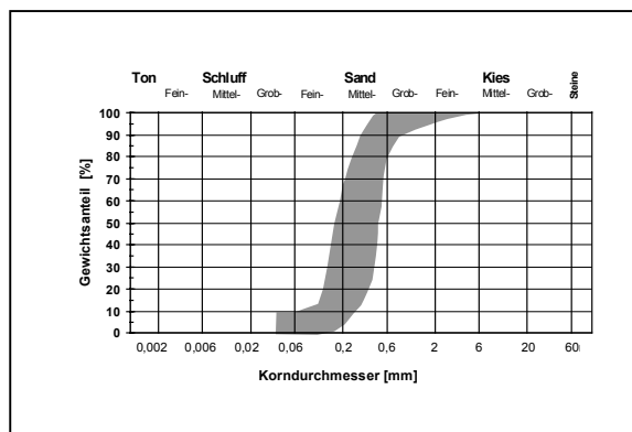
Abb. 9 : Baggerabschnitt 3, Körnungsband Sand (12 Proben)
