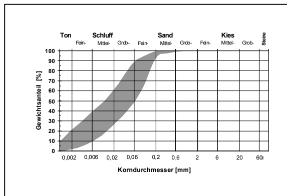
Abb. 8 : Baggerabschnitt 3, Körnungsband Klei (3 Proben)
