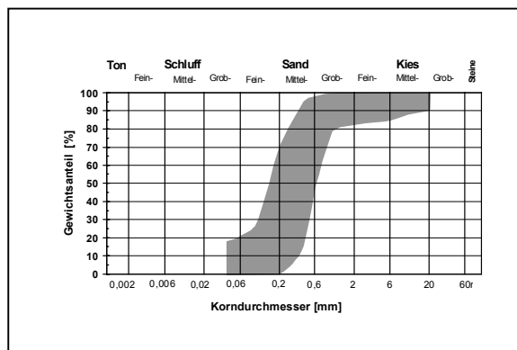
Abb. 7 : Baggerabschnitt 2, Körnungsband Sand (20 Proben)
