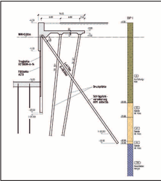
Abb. 1: Konstruktion der Schleusenkammerwand
