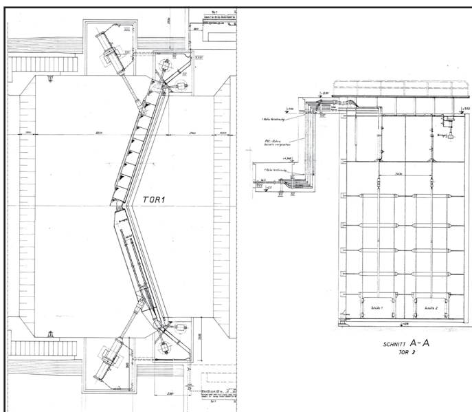
Abb. 1: Grundriss - Ansicht
