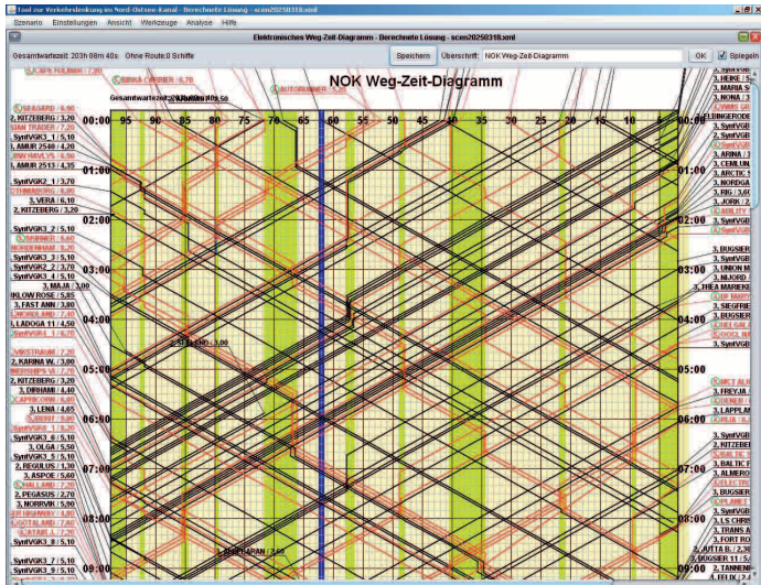
Abb . 5: Verkehr auf dem NOK (Simulation)
