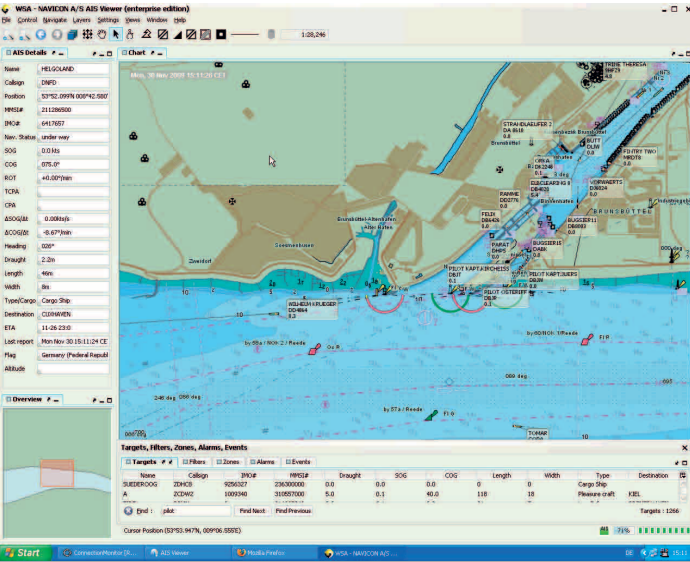
Abb. 2: Bereich Brunsbüttel Zufahrt NOK
