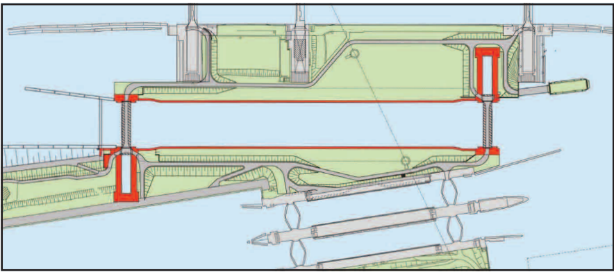
Abb. 2: Zeichnung Neubau 5. Schleusenkammer
