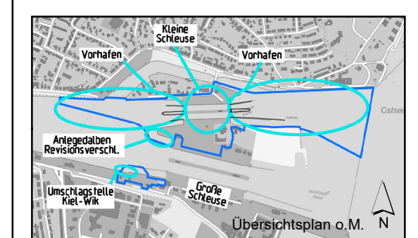
Ersatz der beiden kleinen Schleusenammern und Anpassung der Vorhöfen in Kiel-Holtenauer
