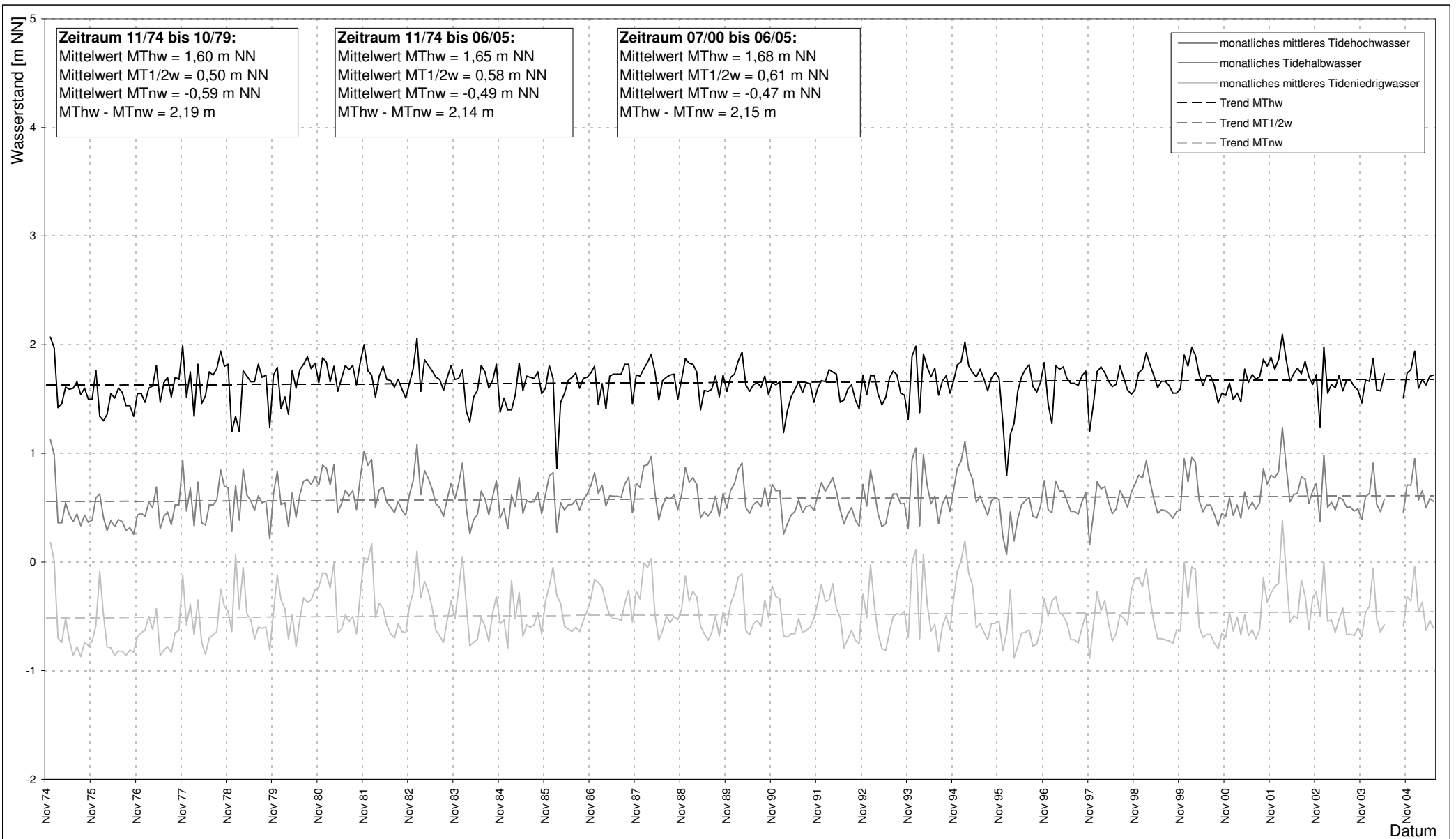
Abb. I-1.5: Monatliche Mittelwerte der Tidewasserstände am Pinnauegel Uetersen von 1974 - 2005
