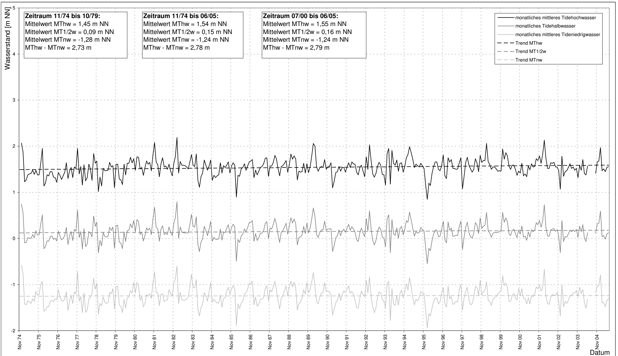
Abb. I-1.1: Monatliche Mittelwerte der Tidewasserstände am Elbpegel Glückstadt von 1974 - 2005
