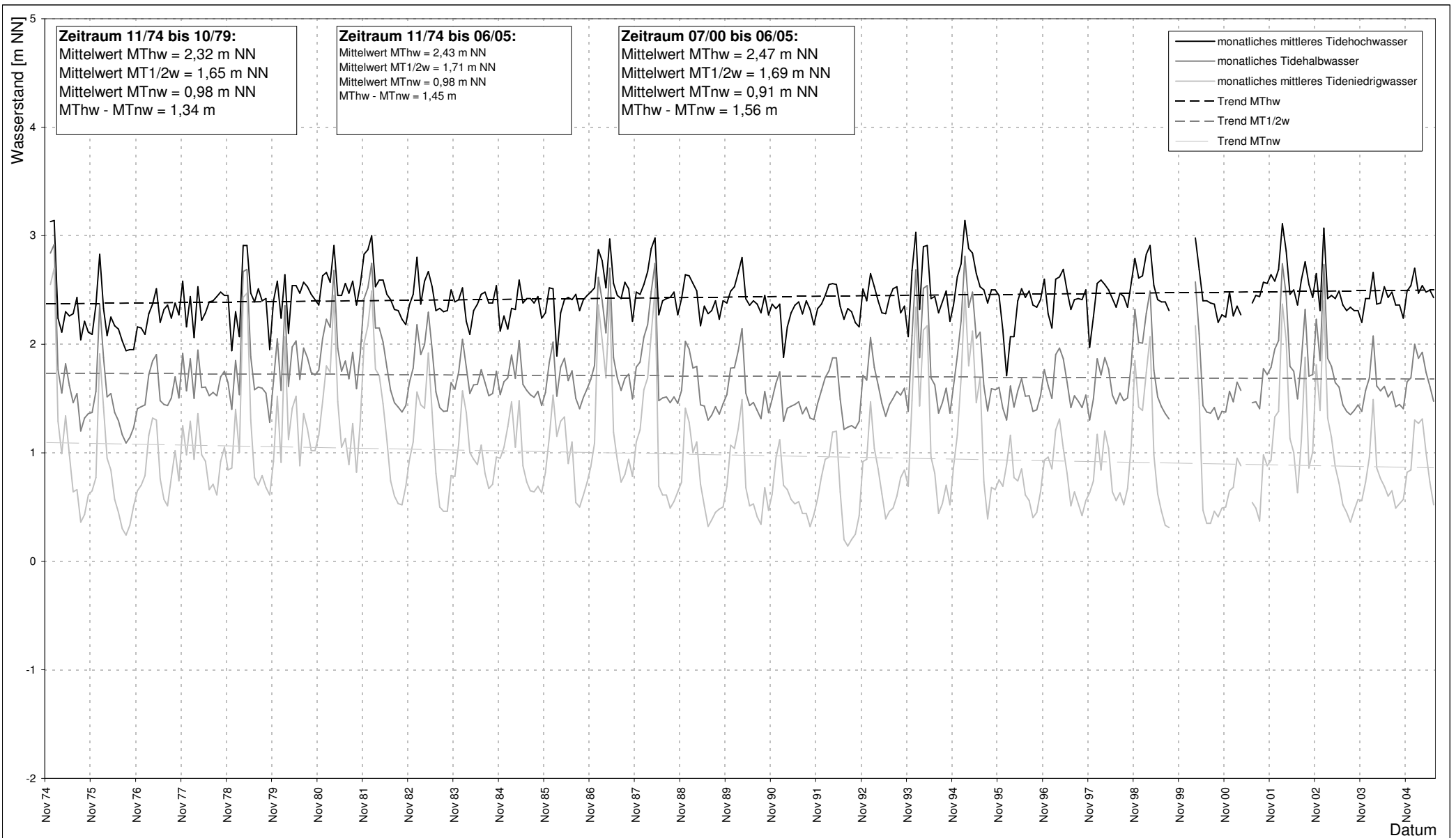
Abb. I-1.7: Monatliche Mittelwerte der Tidewasserstände am Ilmenaupegel Fahrenholz von 1974 - 2005
