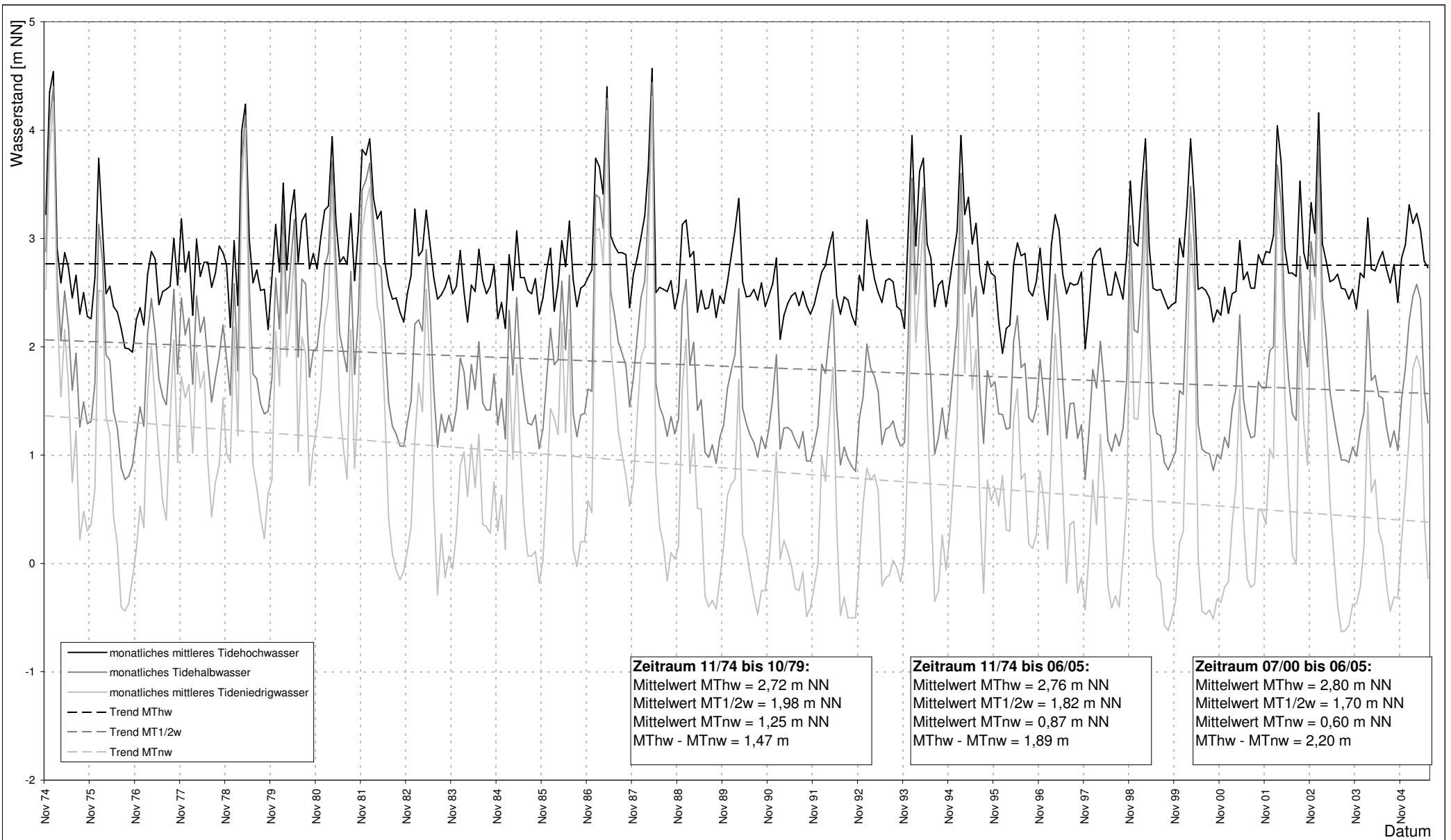
Abb. I-1.3: Monatliche Mittelwerte der Tidewasserstände am Elbpegel Geesthacht von 1974 - 2005
