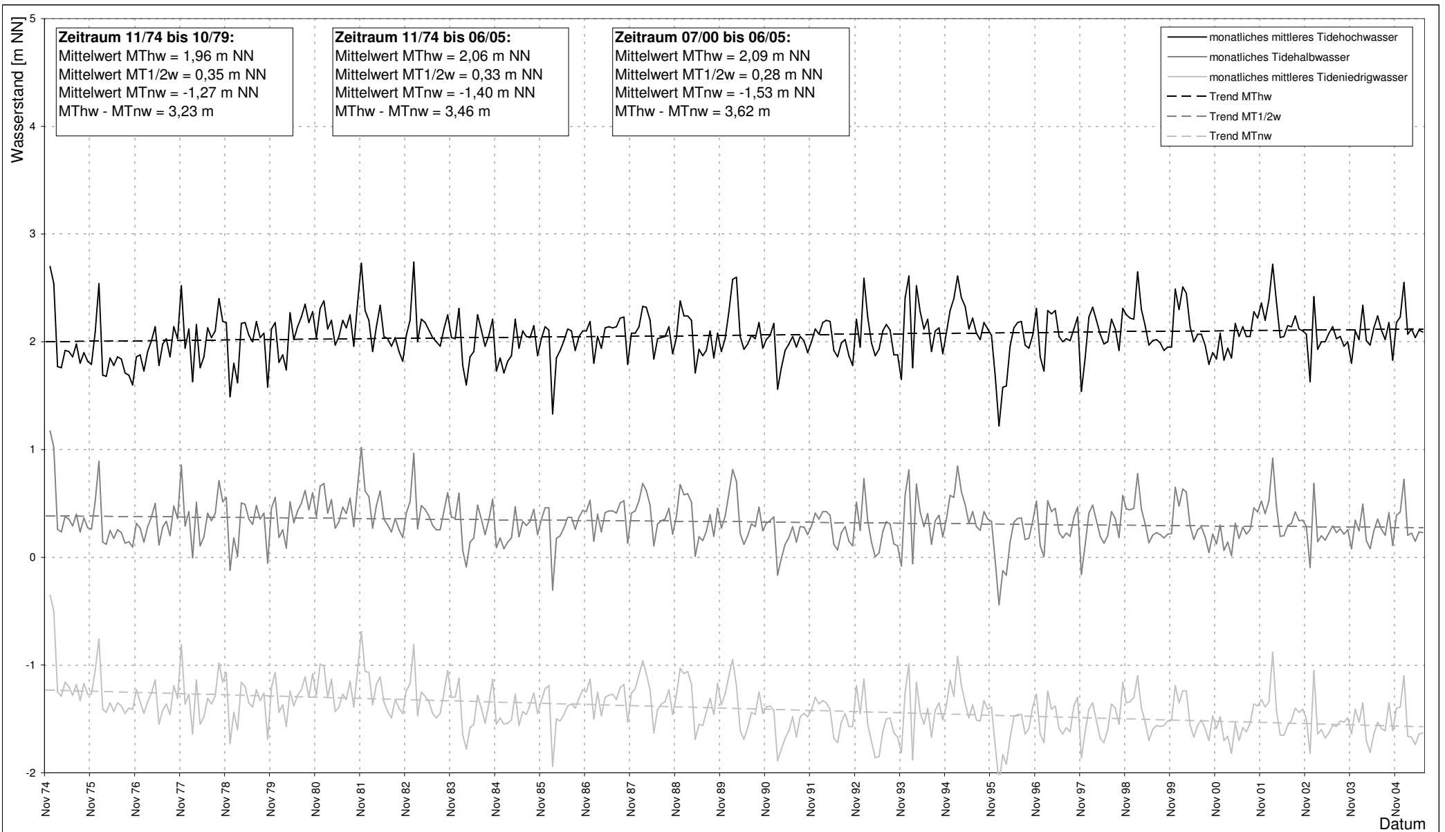
Abb. I-1.2: Monatliche Mittelwerte der Tidewasserstände am Elbpegel St. Pauli von 1974 - 2005
