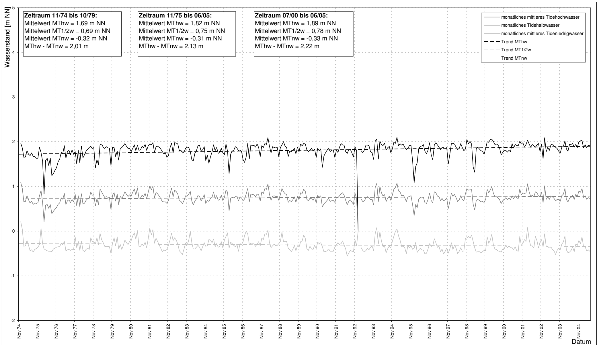
Abb. I-1.6: Monatliche Mittelwerte der Tidewasserstände am Estepegel Buxtehude von 1974 - 2005
