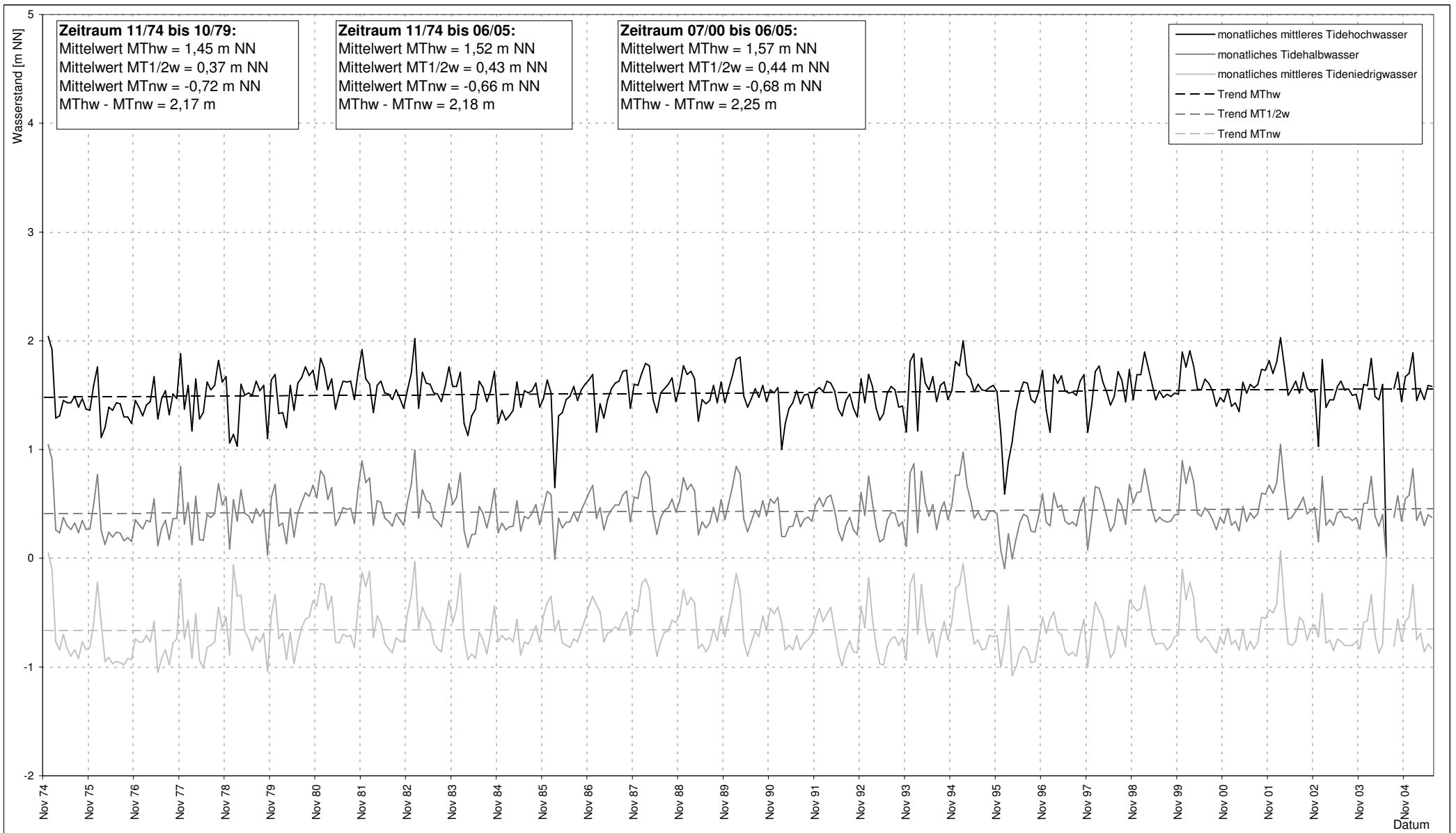
Abb. I-1.4: Monatliche Mittelwerte der Tidewasserstände am Störpegel Itzehoe von 1974 - 2005
