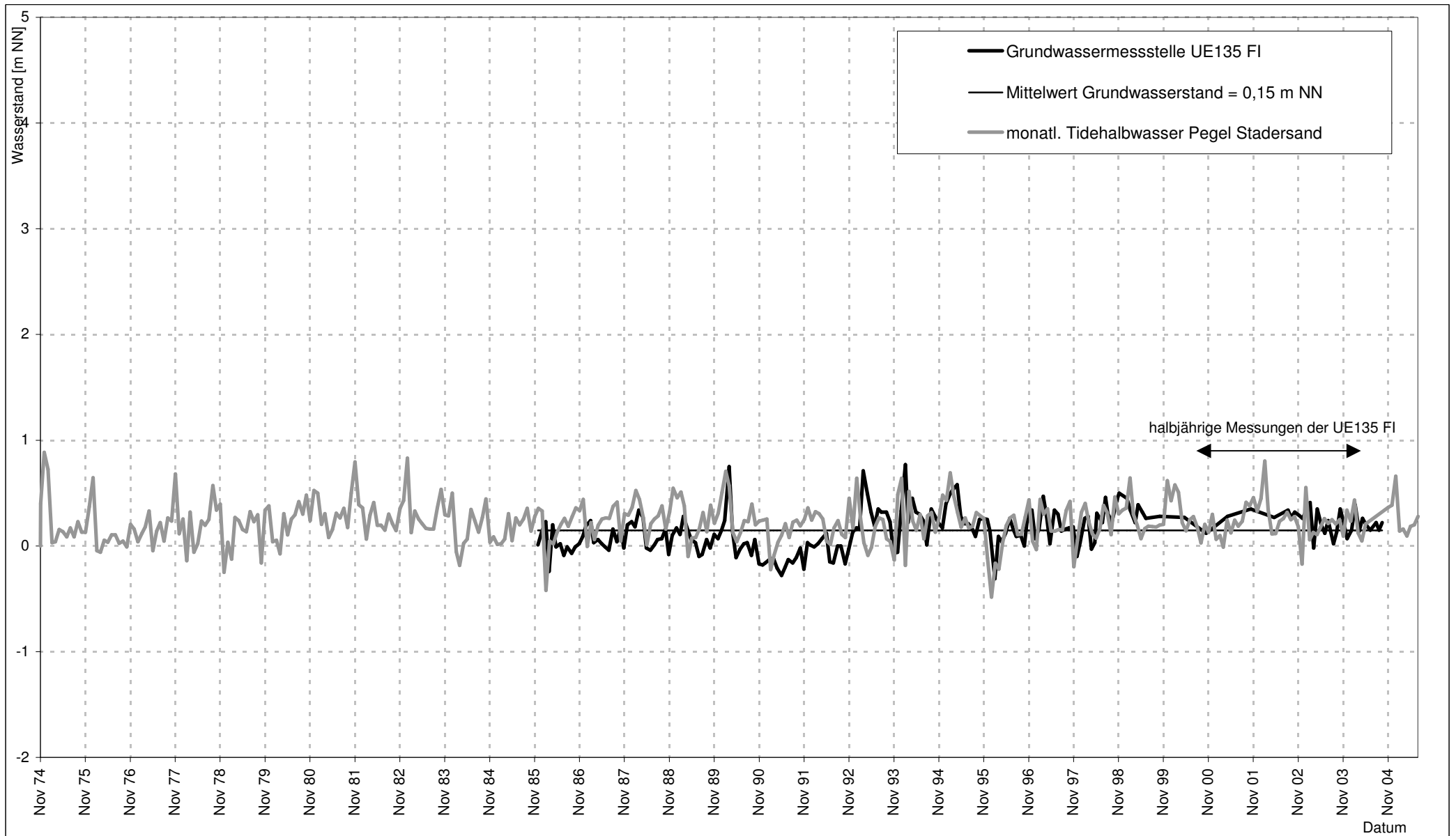
Abb. I-3.1: Grundwasserstände der Messstelle UE135 FI mit Elbeinfluss und Elbwasserstand des Pegels Stadersand; 1974 - 2005 (jeweils Monatsmittelwerte)
