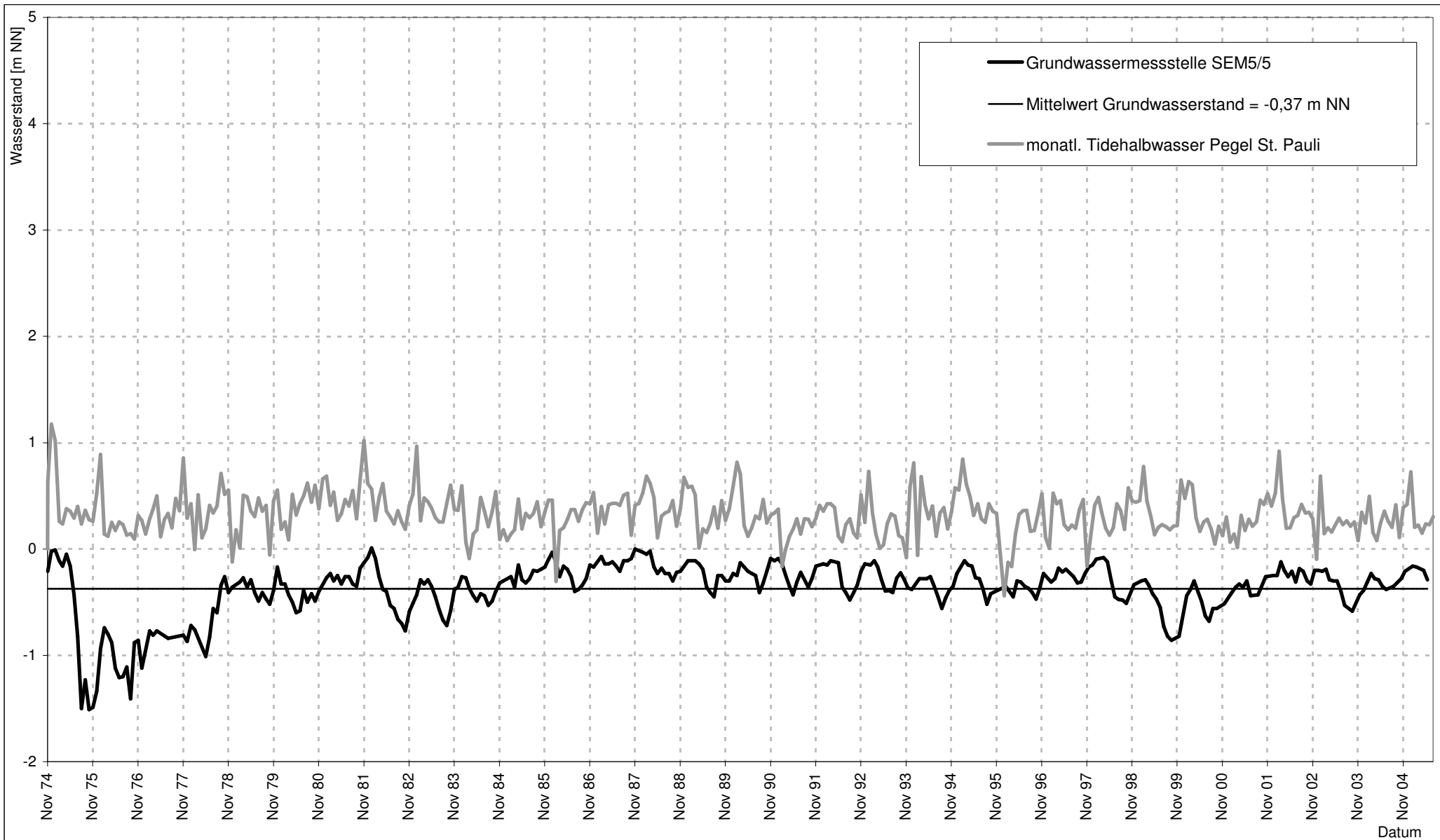
Abb. I-3.3: Grundwasserstände der Messstelle SEM5/5 mit Fördereinfluss und Elbwasserstand des Pegels St. Pauli; 1974 - 2005 (jeweils Monatsmittelwerte)
