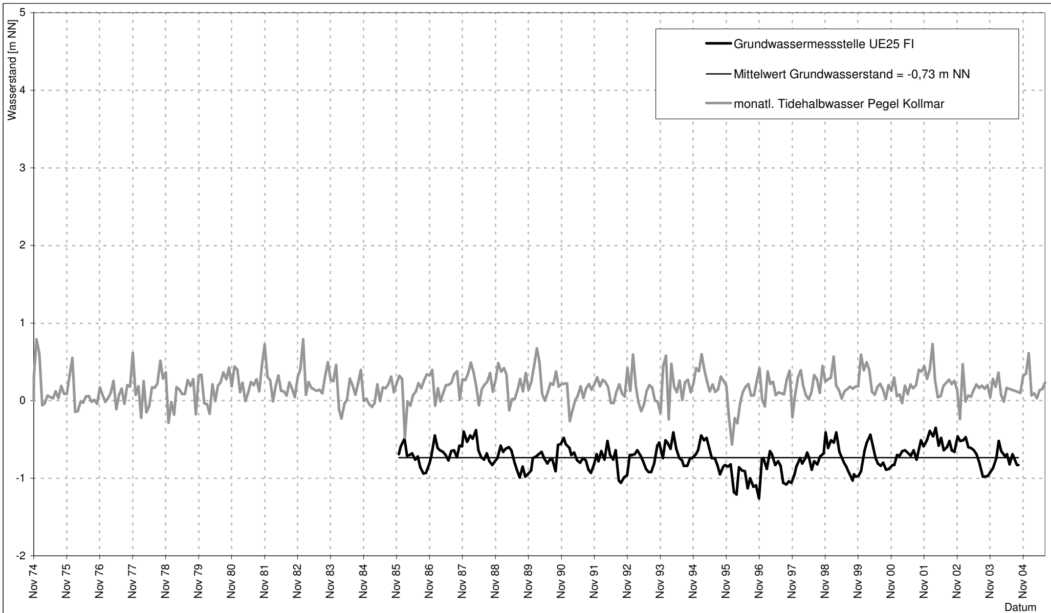
Abb. I-3.2: Grundwasserstände der Messstelle UE25 FI mit Einfluss durch Wasserhaltungsmaßnahmen und Elbwasserstand des Pegels Kollmar; 1974 - 2005 (jeweils Monatsmittelwerte)
