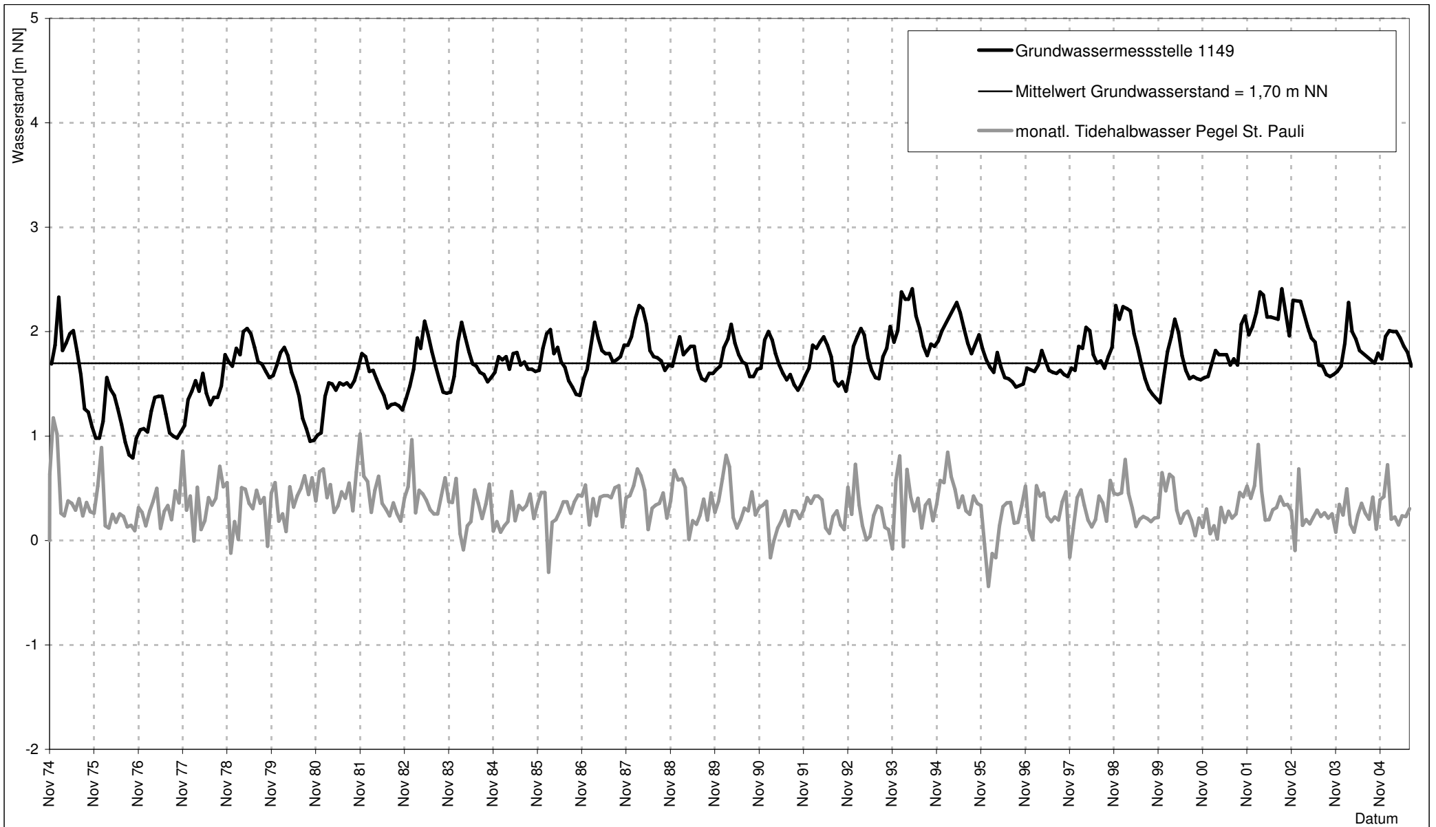
Abb. I-3.4: Grundwasserstände der Messstelle 1149 mit Einfluss durch Niederschlag und Elbwasserstand des Pegels St. Pauli; 1974 - 2005 (jeweils Monatsmittelwerte)
