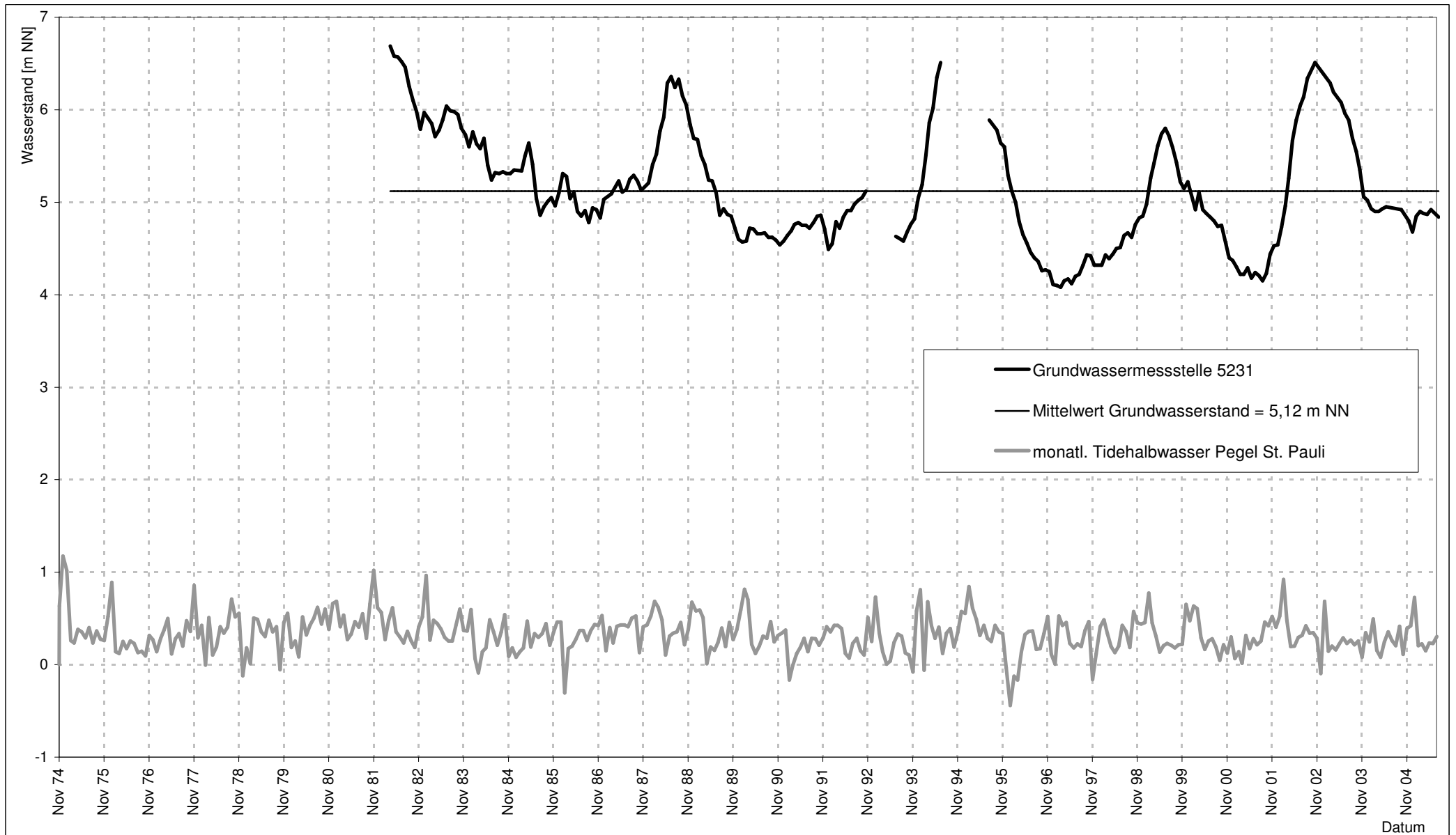
Abb. II-hG14-2: Grundwasserstände der Messstelle 5231 und Elbwasserstand des Pegels St. Pauli; 1974 - 2005 (jeweils Monatsmittelwerte)
