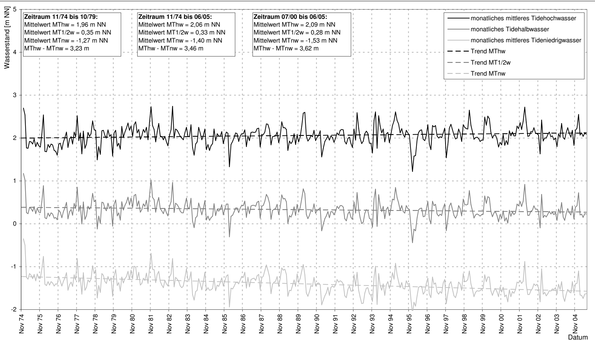
Abb. II-hG14-1: Monatliche Mittelwerte der Tidewasserstände am Elbpegel St. Pauli von 1974 - 2005
